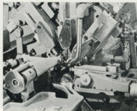
調速軸を作るピーターマン
