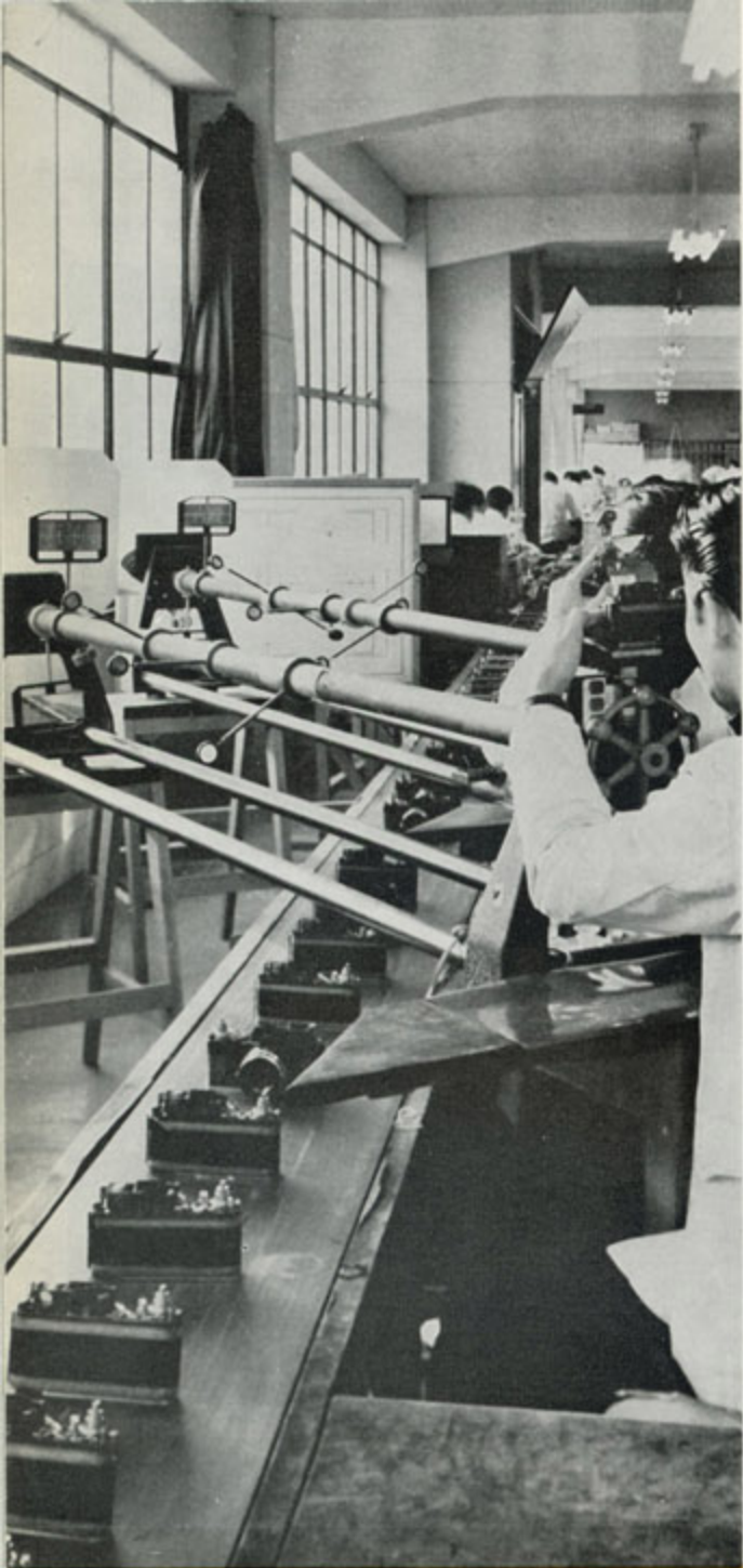
パララックスきょう正検査中
